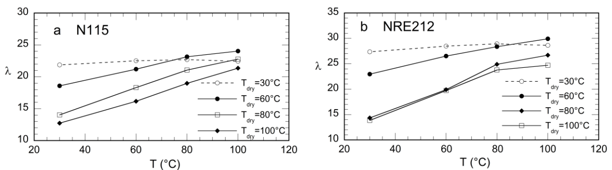
Figure 23. Influence de la température de séchage sur la capacité de sorption des membranes Nafion N115 et NRE212 dans l'eau liquide. Figure issue de la référence [116].
