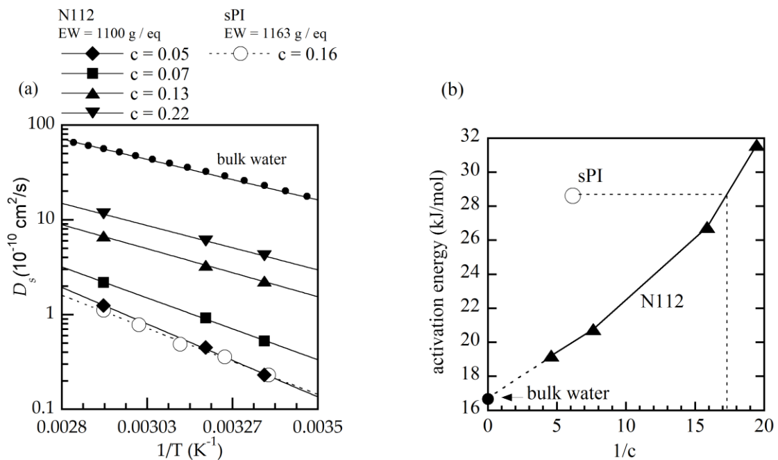
Figure 21. a) Tracé d'Arrhenius du coefficient de diffusion de l'eau dans le Nafion 112 à différentes hydratations et du sPI à c = 0,16 . Les données pour l'eau bulk sont celles de Holz [41]. b) Energies d'activation extraites de a) et tracées en fonction de l'inverse de la fraction massique d'eau.
