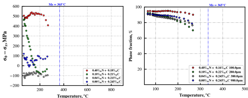
Figure 2: Echantillon nitruré, expérience in situ. Evolutions en fonction de la température en 4 positions dans le gradient a) contraintes dans les phases ferritiques et martensitiques b) fractions massiques des phases ferritiques et martensitiques.
