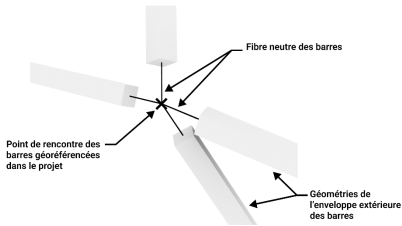
Figure 58. Description géométrique des barres assemblées à un point de rencontre par un nœud d'assemblage
