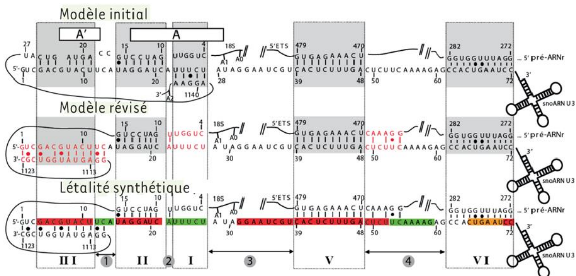
Figure 13 : Appariement entre le snoARN U3 et le pré-ARN ribosomique 35S. Le modèle initial anticipait l'existence de 5 hélices intermoléculaires I, II, III, V et VI, séparées par les segments inter-hélices 1 à 4. Un modèle révisé, issu des données récentes obtenues par cryomicroscopie électronique, ont suggéré l'existence d'une hélice V étendue, l'absence d'hélice I et une hélice III formée avec une autre séquence du pré-ARN 18S (Modèle révisé en rouge). Nos expériences de mutagenèse du snoARNU3 confortent ce nouveau modèle, tandis que les résultats de synthétique létalité réalisés avec le mutant de Rrp9 indique son rôle crucial pour la formation et/ou la stabilisation des hélices II, III et V (Létalité synthétique en rouge) et VI dans une moindre mesure (orange). Les régions non affectées en présence du mutant de Rrp9 apparaissent en vert.
