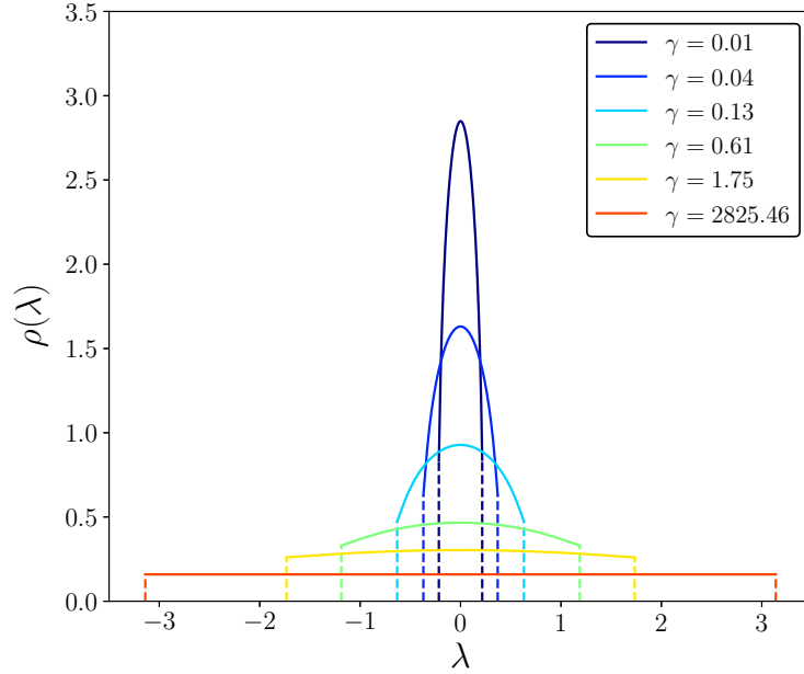
FIGURE 2.2 – La distribution de rapidité pour différentes valeurs de \gamma . À mesure que la force d'interaction augmente, la densité de rapidité s'étale pour devenir finalement constante sur son domaine de définition quand \gamma \rightarrow \infty . Cette figure est une reproduction de la figure 2 de la référence [1]
