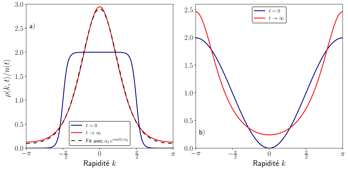
FIGURE 7.3 – Comportement aux temps longs du rapport \rho(k, t)/n(t) pour différentes distributions initiales. a) En bleu, la distribution initiale prise comme une distribution de Fermi-Dirac \rho_0(k) = (1 + \exp(-\cos(k)/T))^{-1} avec une température T=0.1 . En rouge, l'allure de la distribution quand t \rightarrow \infty obtenue avec la solution analytique (7.48). La courbe en pointillés noirs représente un fit numérique avec une distribution de Boltzmann a_1 \exp\{\cos(k)/a_2\} . b) En bleu, la distribution initiale prise comme une distribution non thermique \rho_0(k) = (1 - \cos(sk))/2 . En rouge la distribution à des temps infinis. Cette dernière est clairement incompatible avec état thermique.
