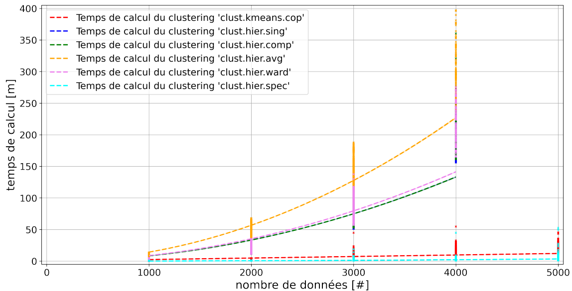
FIGURE 4.17 – Estimation du temps nécessaire (en minutes) pour effectuer une tâche de clustering en fonction du nombre de données à traiter.
