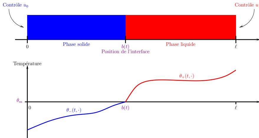
FIGURE 1.4 – Représentation schématique du problème de Stefan à deux phases.
